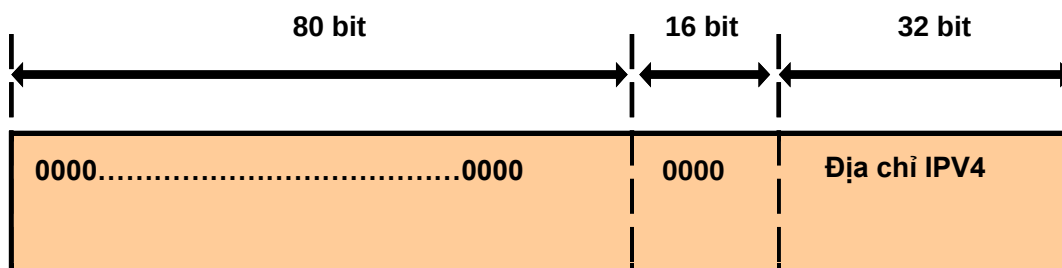
Hình 13: Địa chỉ IPv4-compatible
