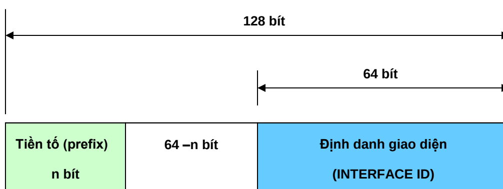
Hình 6: Cấu trúc thường thấy của một địa chỉ IPv6
