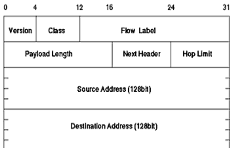
Hình 22: IPv6 header
