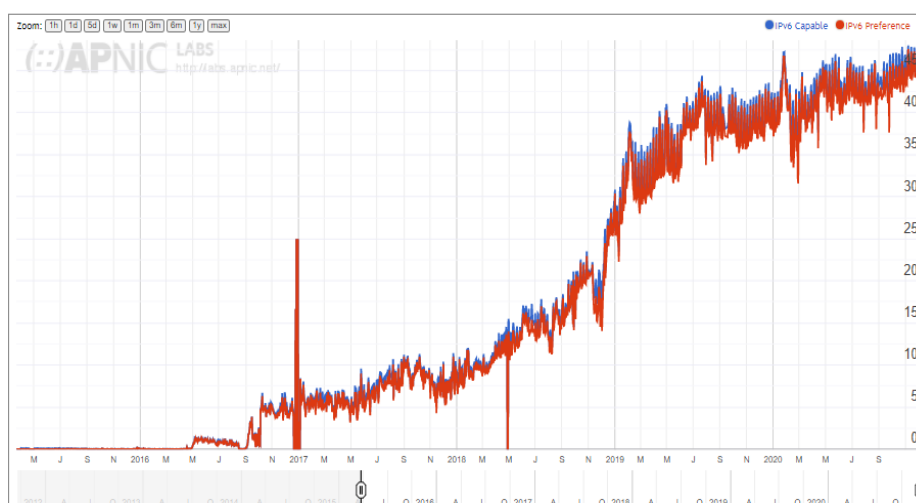
Hình 5: Tỷ lệ ứng dụng IPv6 Việt Nam (tháng 12/2020, nguồn APNIC)
