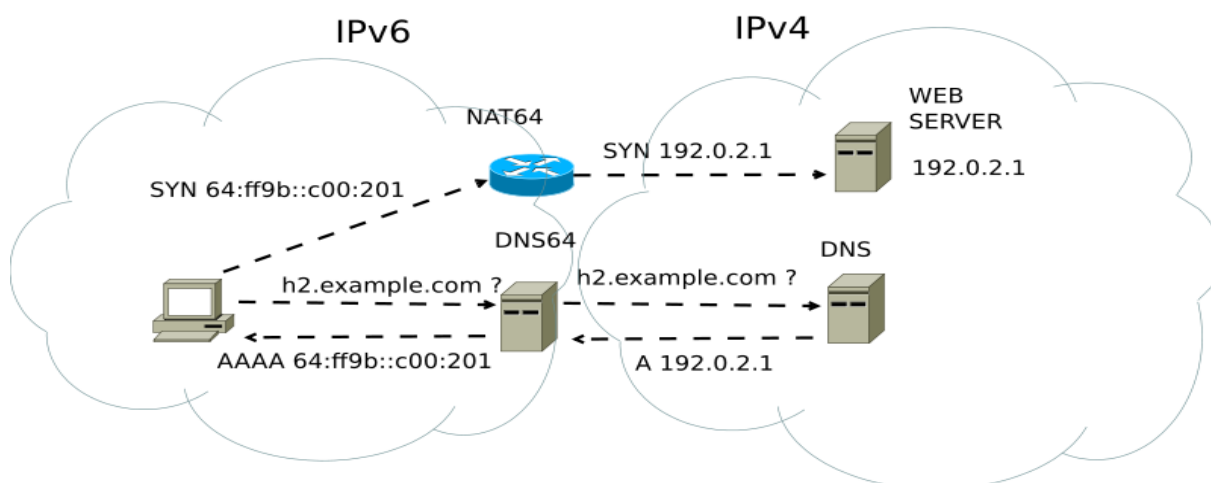
Hình 36: Công nghệ biên dịch
