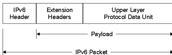
Hình 23: Cấu trúc gói tin IPv6
