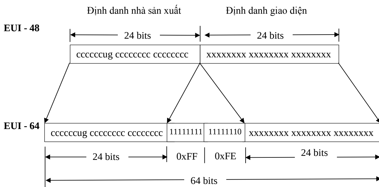
Hình 7: Ánh xạ từ EUI-48 tới EUI-64
