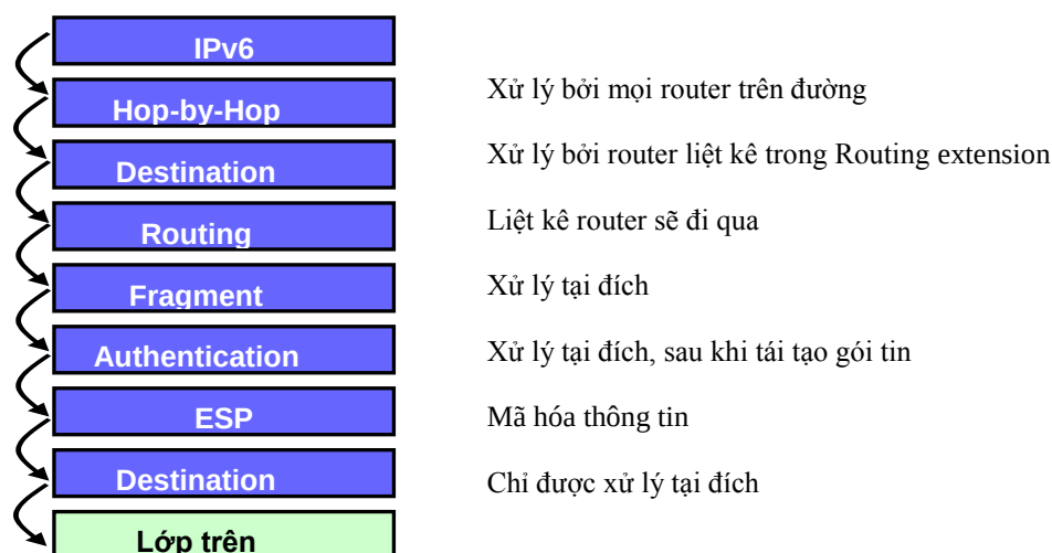
Hình 25: Thứ tự xử lý các header mở rộng
