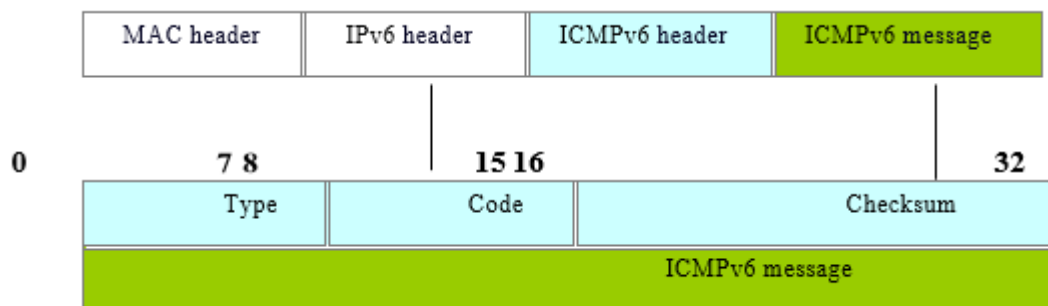
Hình 28: Cấu trúc gói tin ICMPv6
