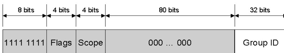
Hình 16: Cấu trúc địa chỉ IPv6 multicast
