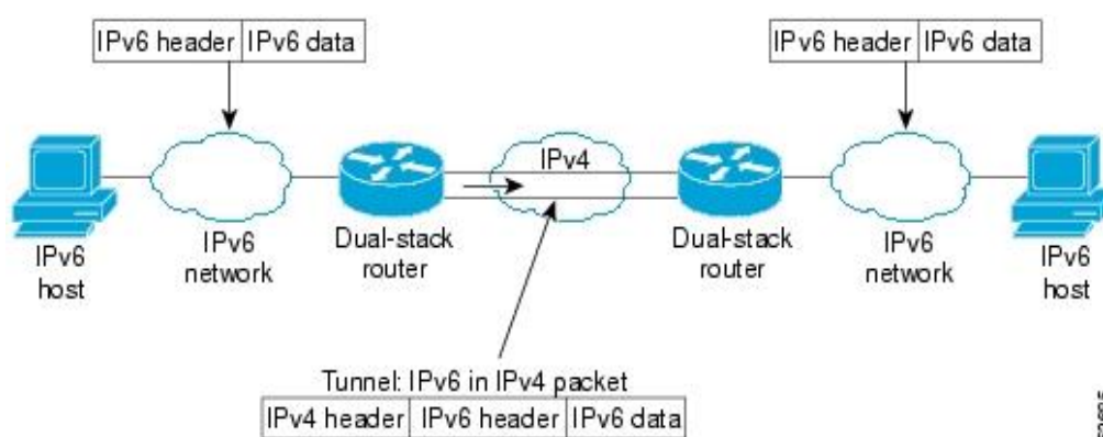
Hình 37: Công nghệ đường hầm
