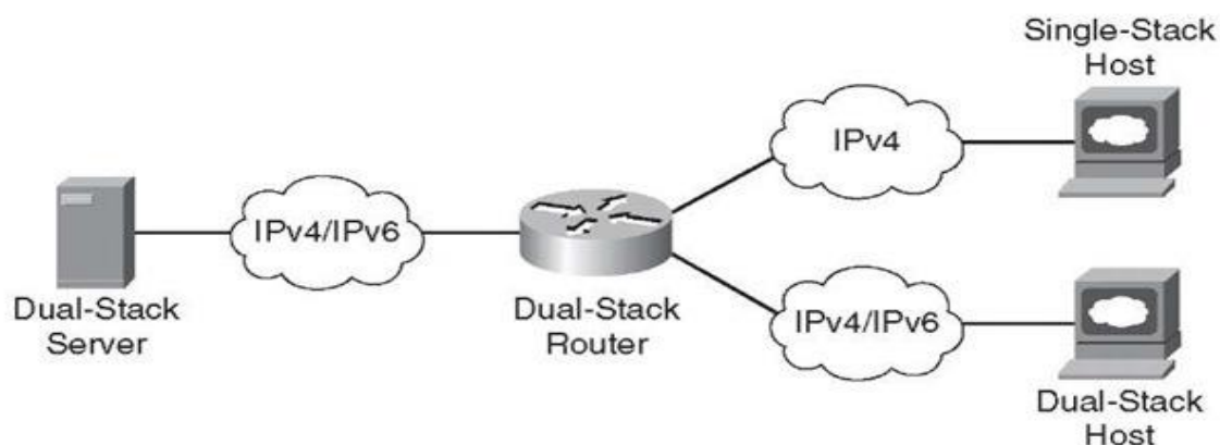
Hình 35: Công nghệ dual-stack
