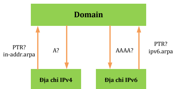
Hình 43: Quy trình truy vấn IPv4, IPv6 trên hệ thống DNS
