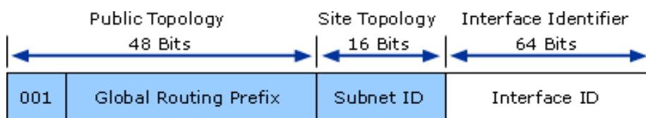
Hình 12: Phân cấp định tuyến địa chỉ IPv6 unicast toàn cầu
