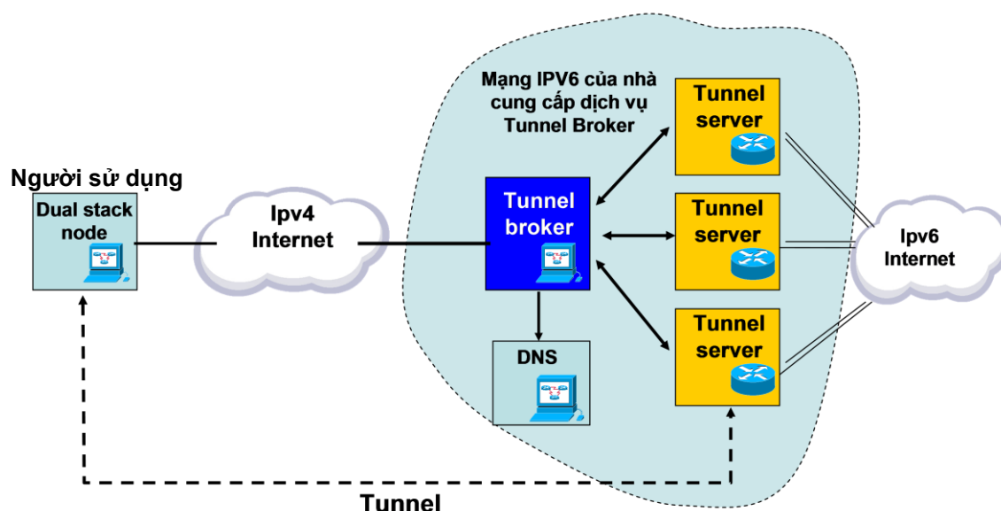
Hình 39: Mô hình của tunnel broker
