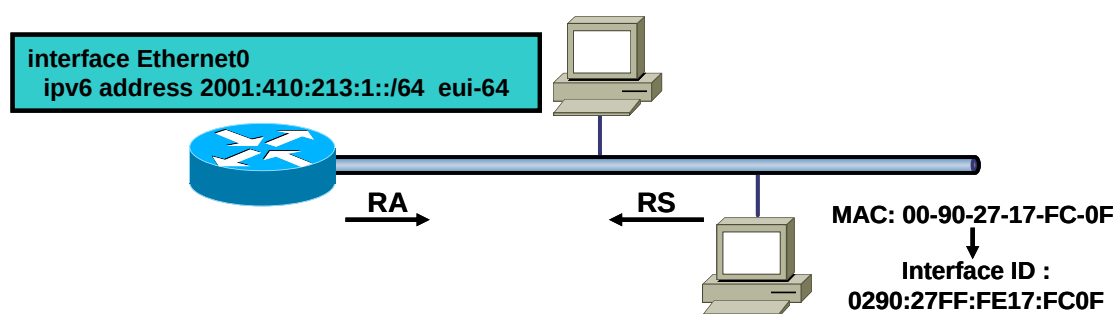
Hình 31: Tự động cấu hình địa chỉ của IPv6 host
