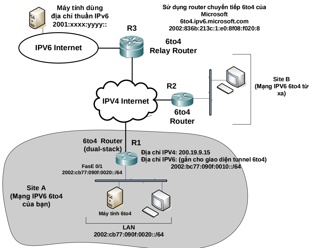
Hình 41: Sử dụng tunnel 6to4 kết nối Internet IPv6
