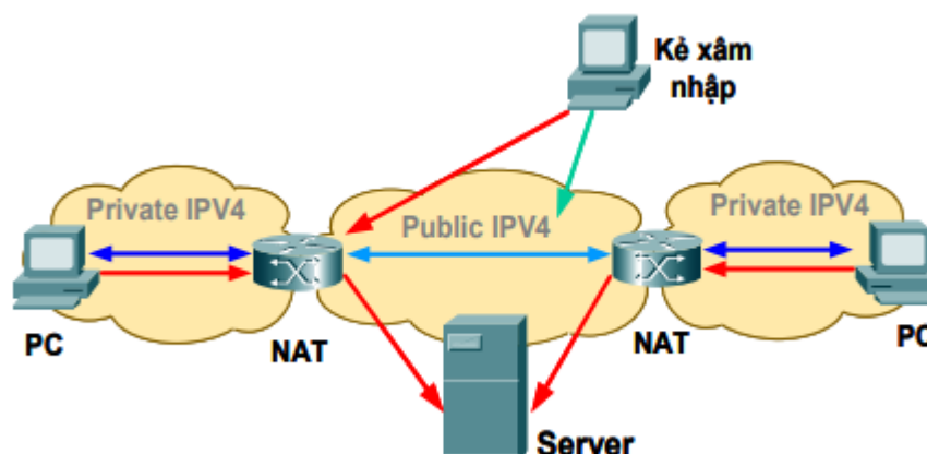
Hình 3: Mô hình thực hiện NAT của địa chỉ IPv4
