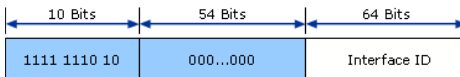
Hình 9: Cấu trúc địa chỉ link-local
