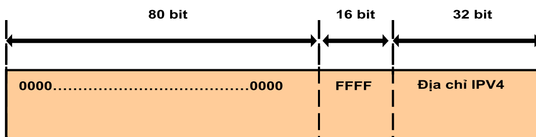
Hình 14: Địa chỉ IPv4-mapped
