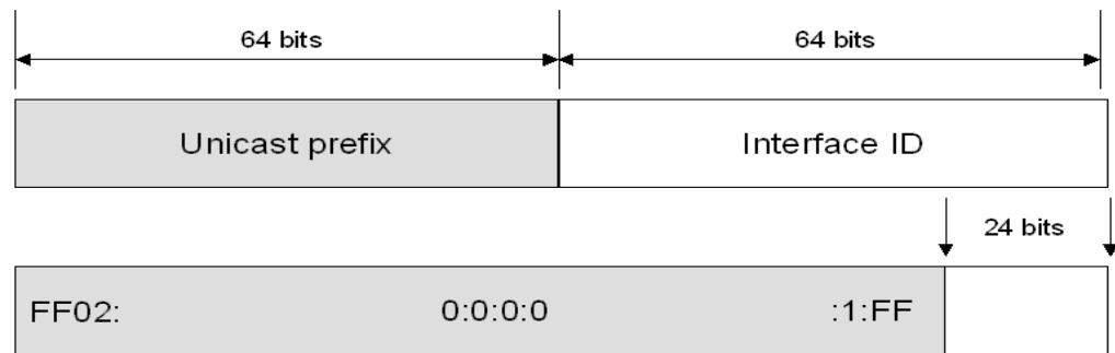
Hình 19: Cấu thành địa chỉ solicited-node multicast từ địa chỉ unicast
