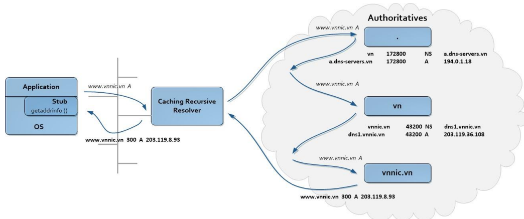
Hình 42: Mô hình hoạt động của hệ thống DNS
