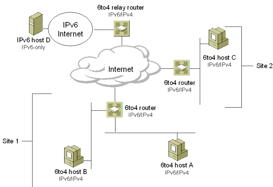
Hình 40: Các thành phần của tunnel 6to4
