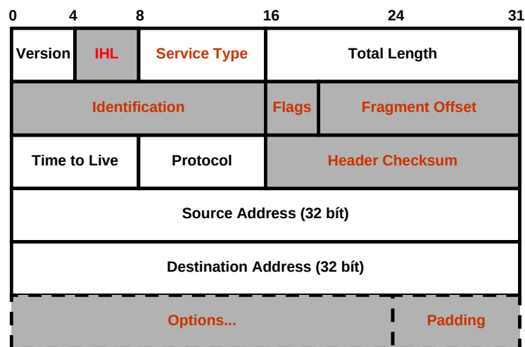
Hình 21: IPv4 header
