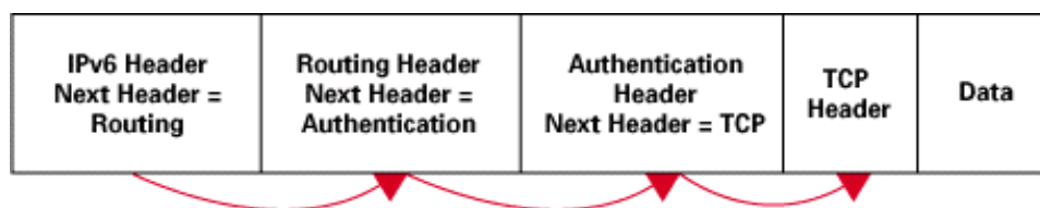
Hình 24: Header mở rộng của địa chỉ IPv6
