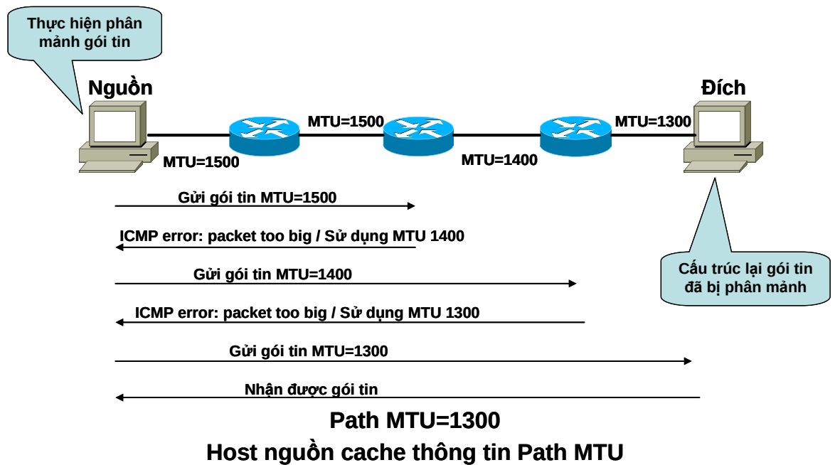
Hình 32: Quy trình thực hiện tìm kiếm Path MTU
