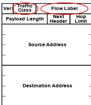
Hình 27: Hỗ trợ QoS trong địa chỉ IPv6
