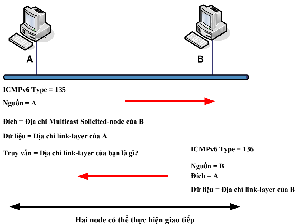
Hình 30: Quy trình phân giải địa chỉ
