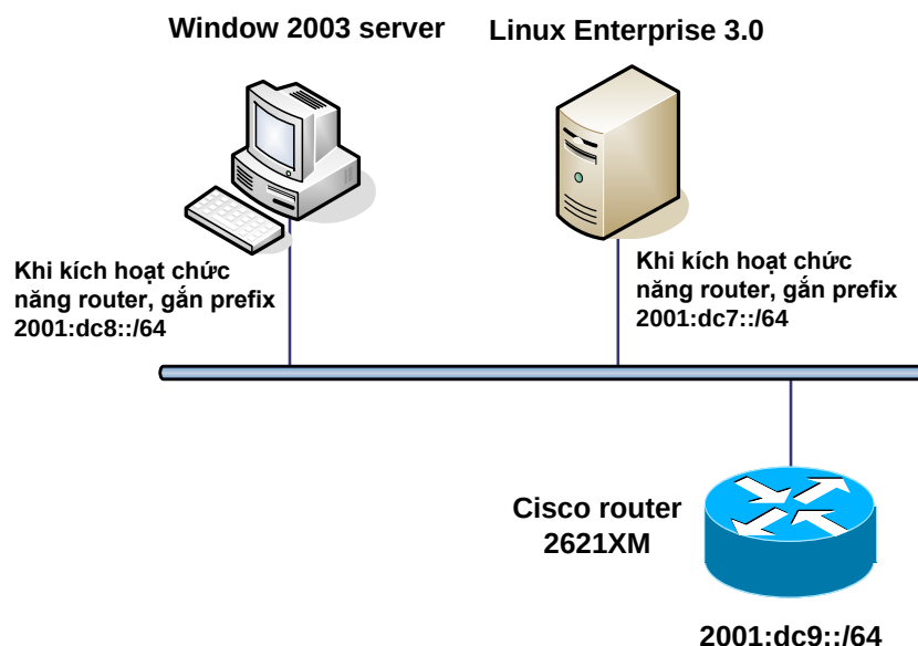
Hình 33: Mạng thực hành
