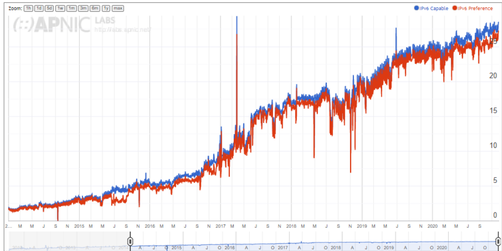
Hình 4: Tốc độ tăng trưởng ứng dụng IPv6 toàn cầu (tháng 12/2020, nguồn APNIC Lab)
