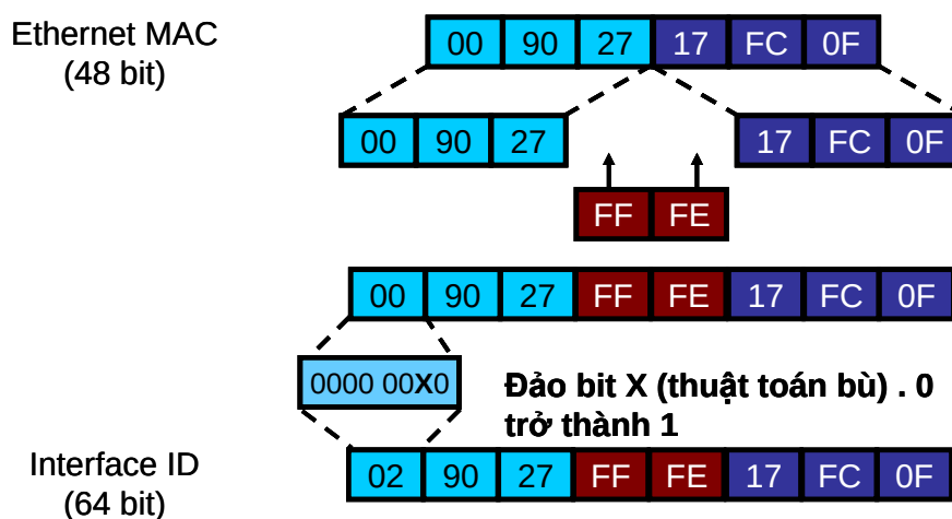
Hình 8: Tự động cấu hình 64 bit định danh giao diện từ địa chỉ MAC
