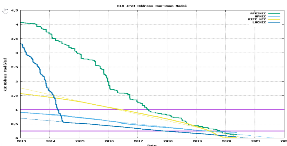
Hình 2: Biểu đồ cạn kiệt địa chỉ IPv4 toàn cầu (nguồn APNIC)
