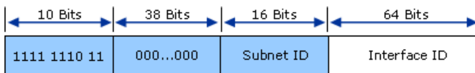
Hình 10: Cấu trúc địa chỉ site-local
