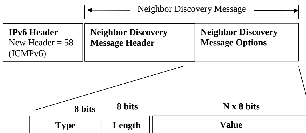
Hình 29: Cấu trúc thông điệp ND
